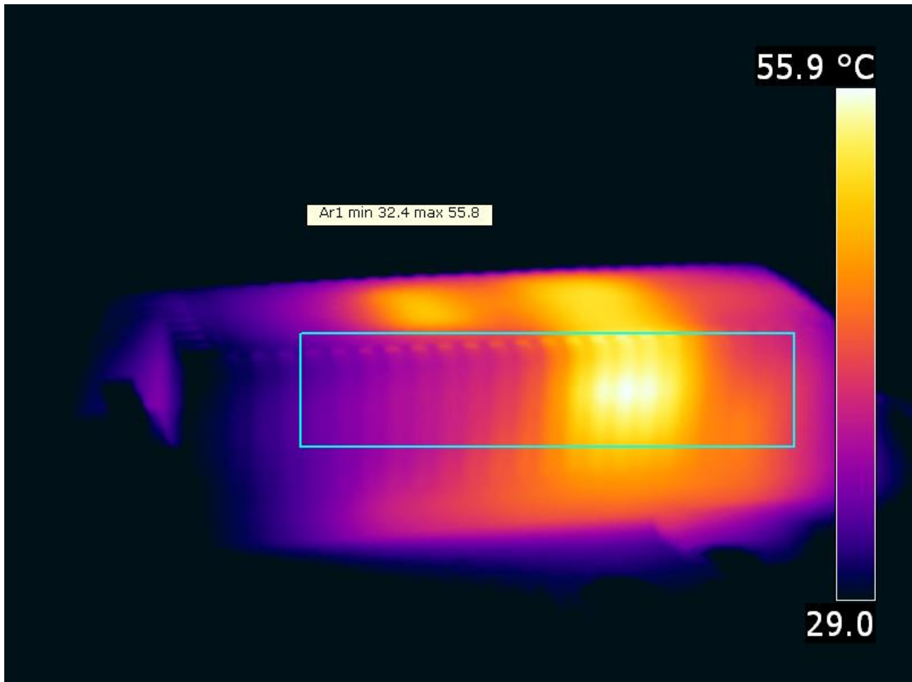
Temperatuurplaatje van de buis en de voeding.
