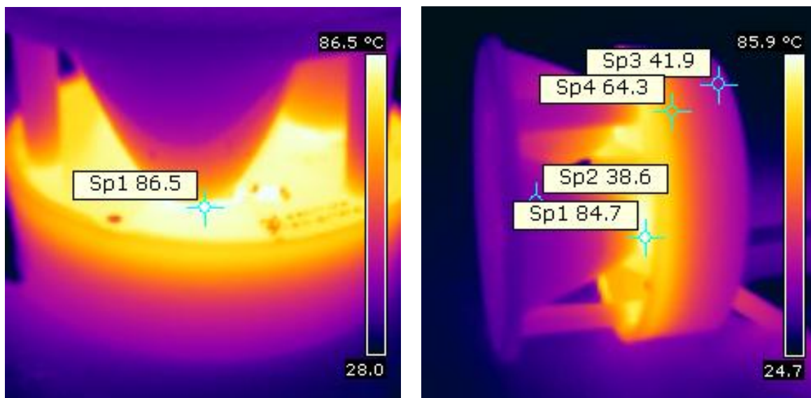
Temperatuursplaatjes van de lamp na opwarmen.
