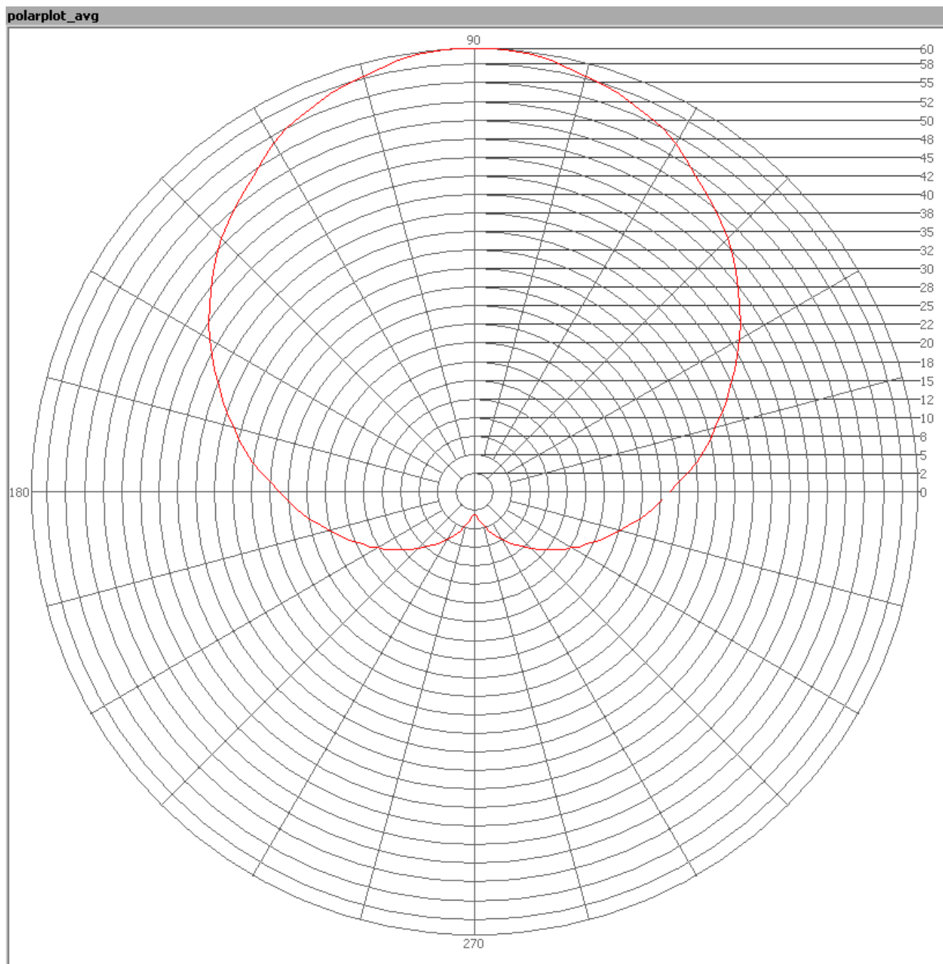
Das Strahlungsdiagramm der Lampe.
