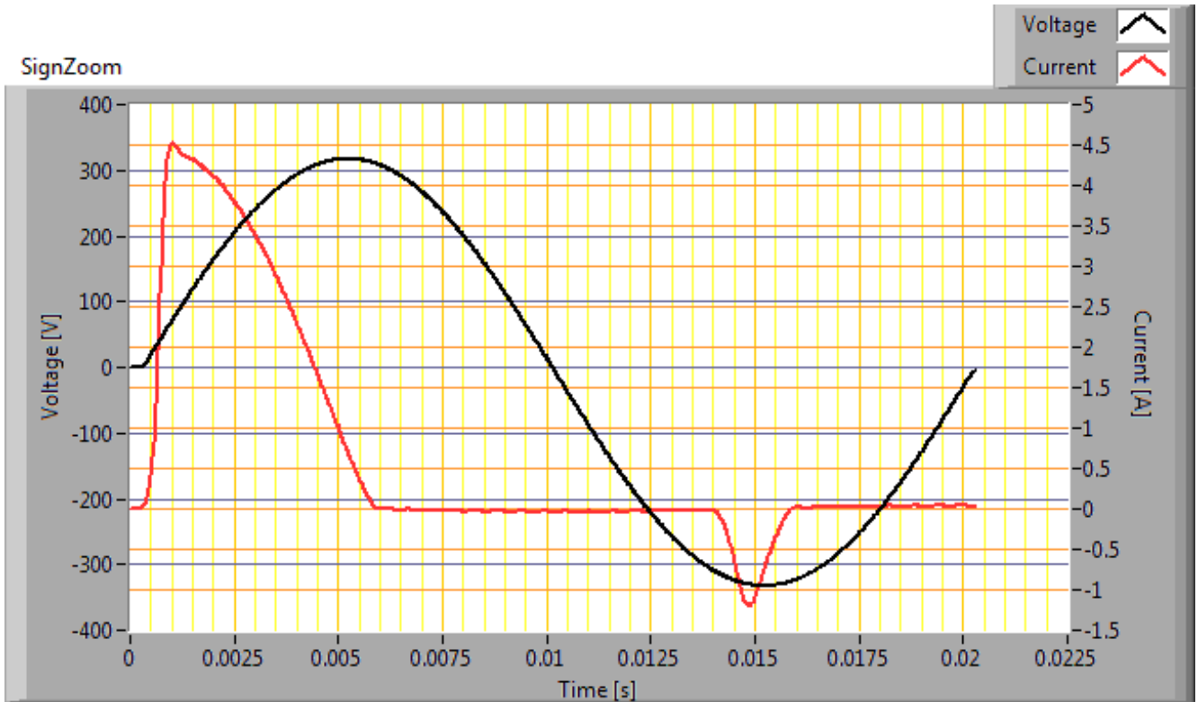
Premier cycle du courant de démarrage
