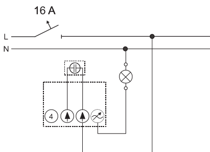
Afb. 2: Standaardgebruik: voor mogelijke belastingtypen zie hoofdstuk "Soort belasting" op pagina 5
